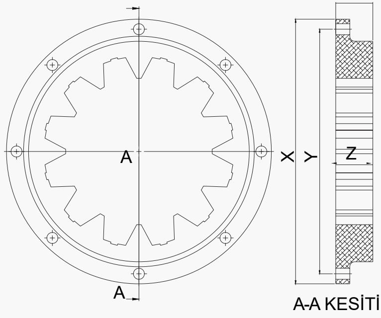
SAE YILDIZ KAPLİN ÖLÇÜLERİ SAE ENGINE FLYWHEEL DIMENSIONS
